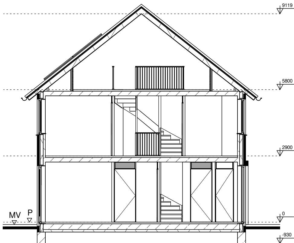
Doorsnede A
